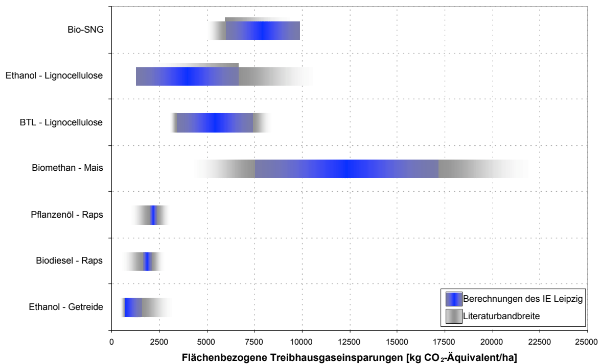
Abb. 5 - Flächenbezogene Treibhausgaseinsparungen
