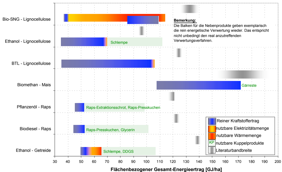
Abb. 3 - Flächenbezogener Gesamt-Energieertrag
