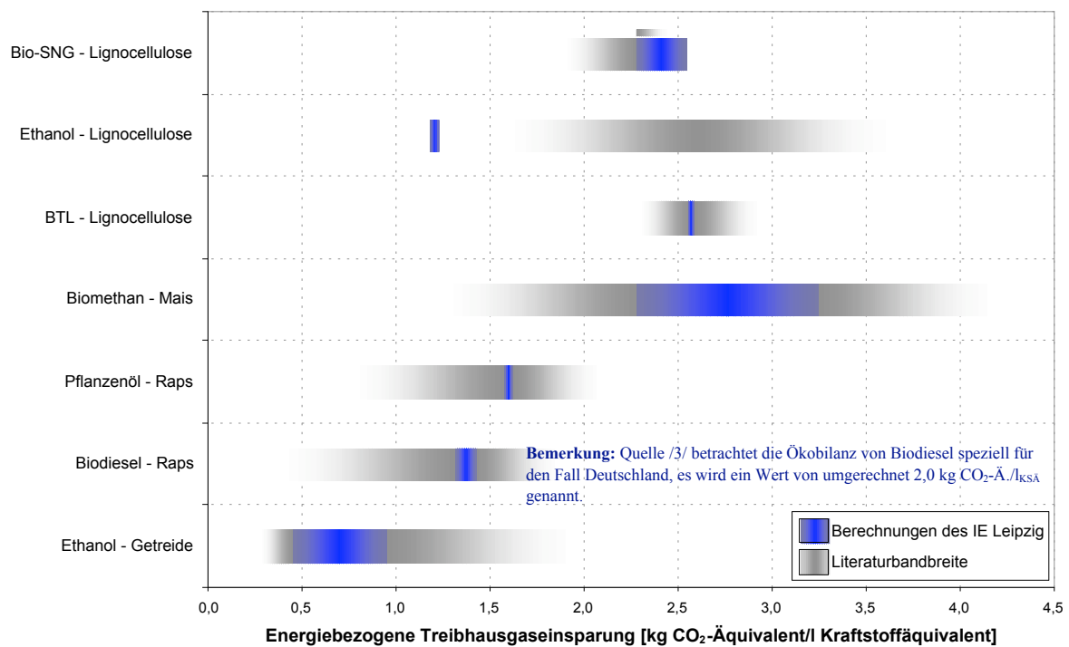
Abb. 4 - Energiebezogene Treibhausgaseinsparung
