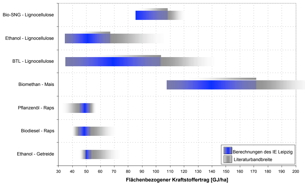
Abb. 2 - Flächenbezogener Kraftstofffertrag
